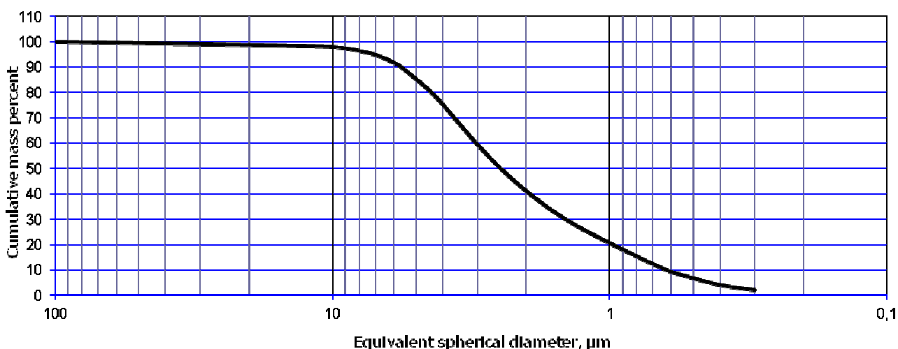
Distribuzione granulometrica / particle size distribution
