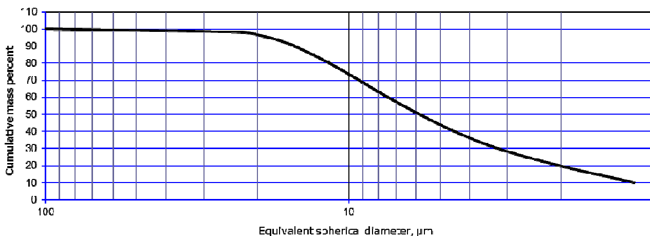
Distribuzione granulometrica / particle size distribution
