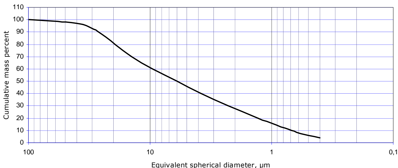
Distribuzione granulometrica / particle size distribution
